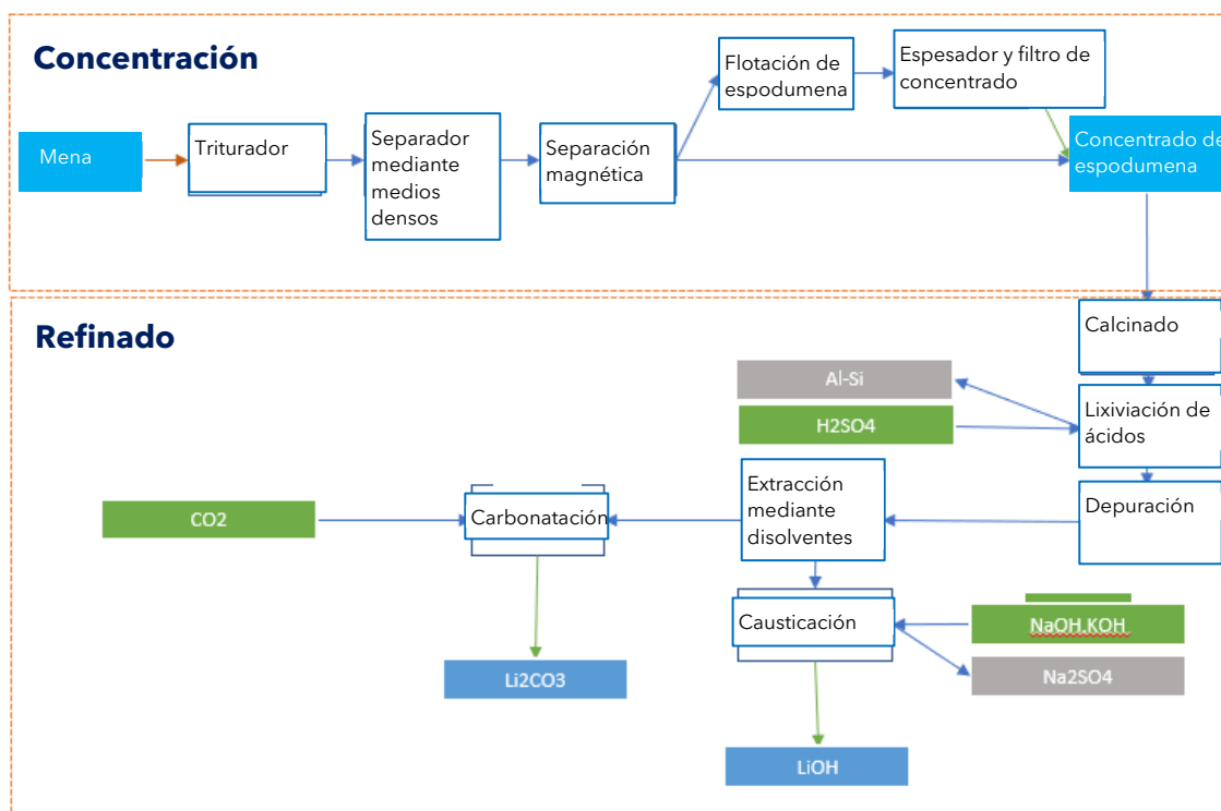
Gráfico 4. Proceso de producción de litio a partir de minerales - Diagrama del proceso
