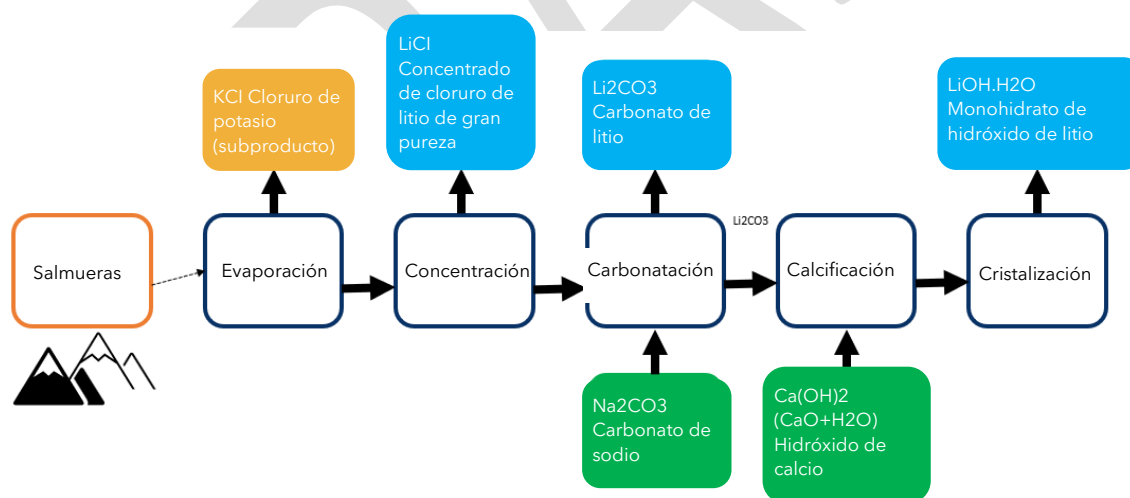
Gráfico 3. El proceso de producción de litio a partir de salmueras - Diagrama del proceso
